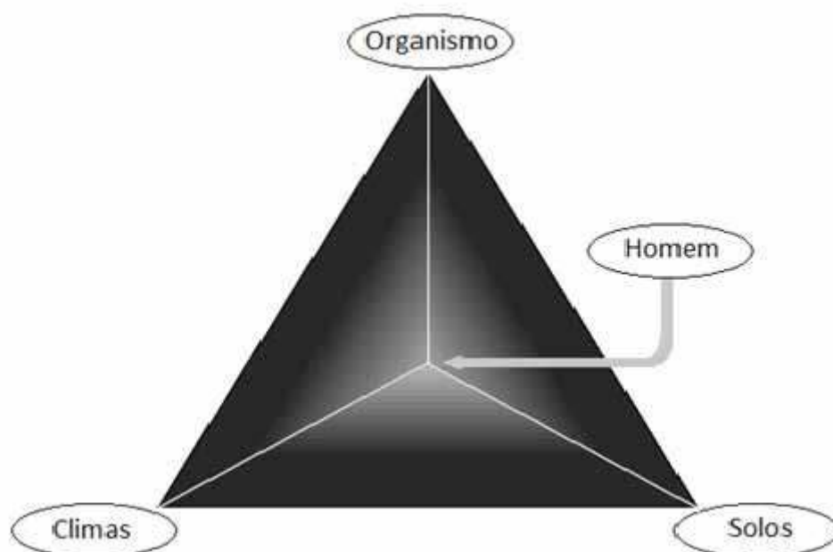
FIGURA 01: Representação do tetraedro ecológico de acordo com Resende, Lani e Feitoza (1993).
