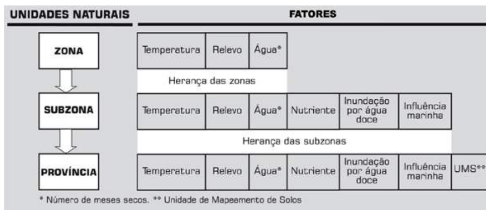
Figura 02: Representação da hierarquia das Unidades Naturais com os fatores que participam de cada nível (FEITOZA, 2001a)
