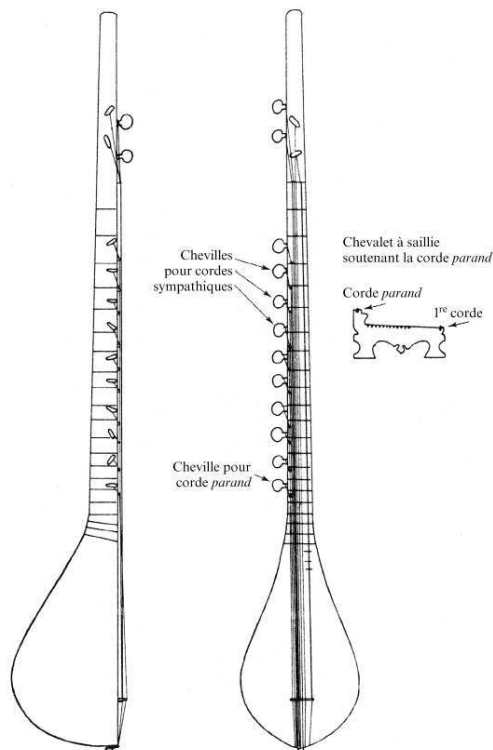
Fig. 1 : Le dutâr à quatorze cordes de Hérat
