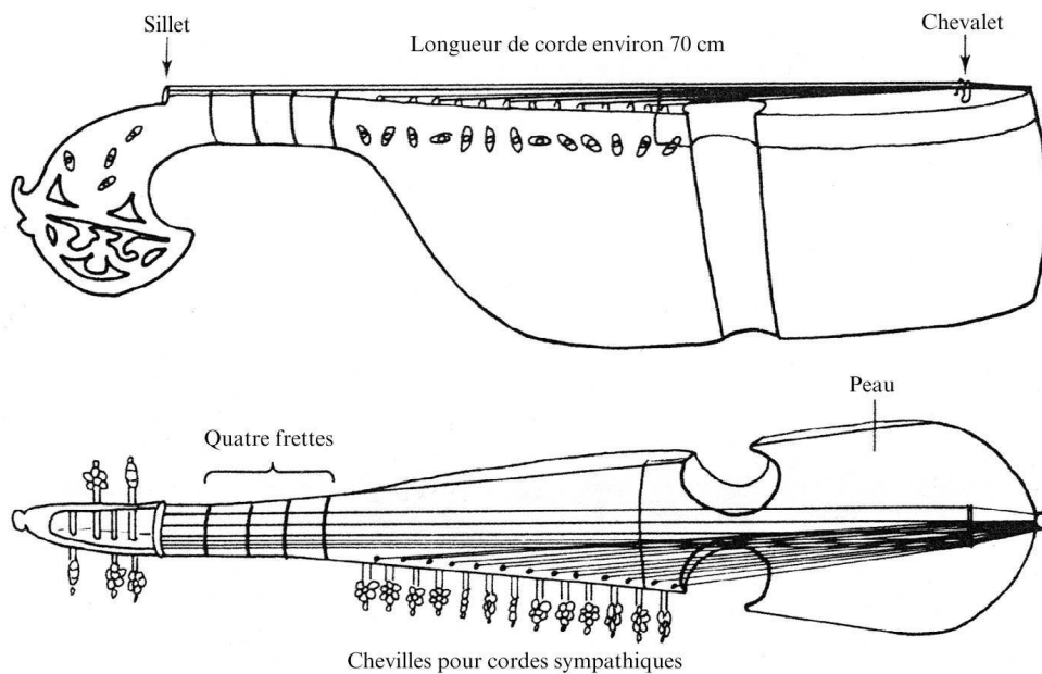
Fig. 2 : Le rubâb afghan
